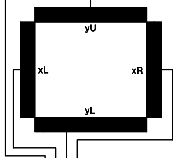
Touch Panel Pin-assign (Pin-assign from Touch side) (タッチパネル ピンアサイン。 タッチ面側からのピンアサイン)
